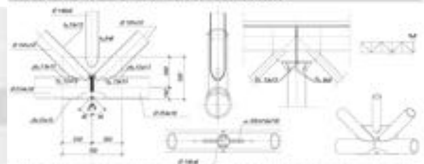
FIG. 21.112. RIGHE INALZATE E DIMENSIONI IN ALZATE PER PROFILI A SEZIONE CAVA.
